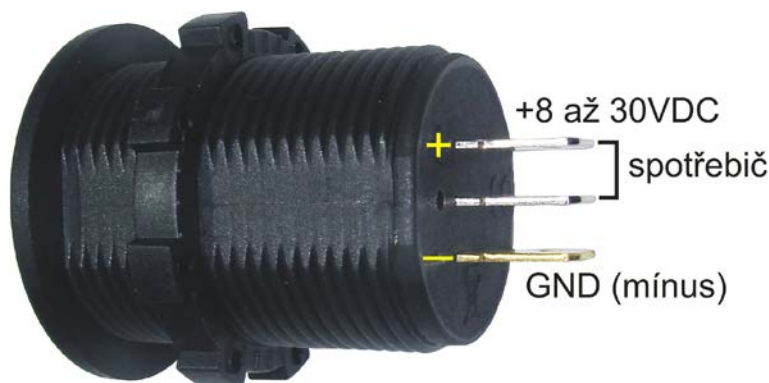
Připojení k napájecímu napětí a spotřebiče
